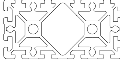
90x180Z Art 222013
